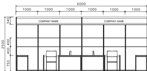
ELEVATION 正面圖
