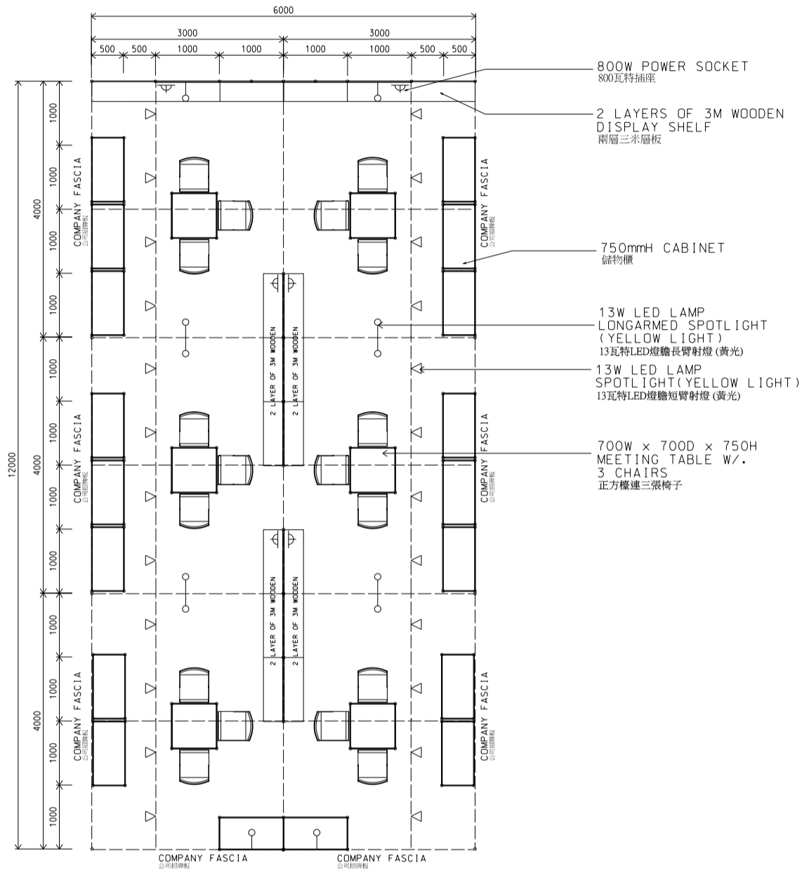
PLAN 平面圖
