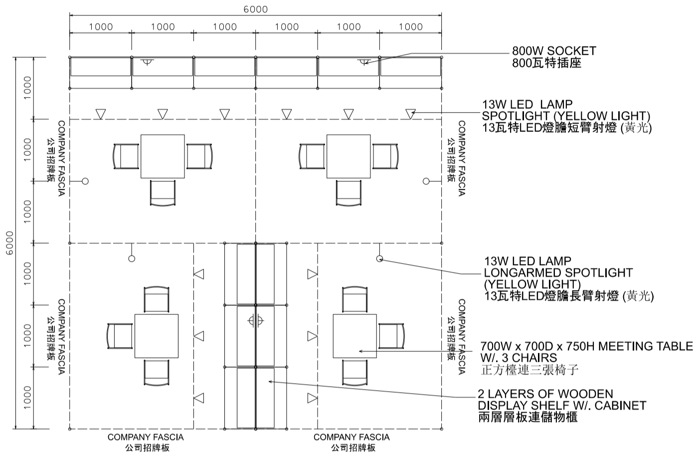
PLAN 平面圖
