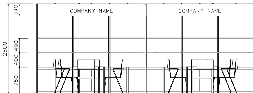
ELEVATION 正面圖
