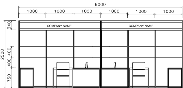
ELEVATION 正面圖
