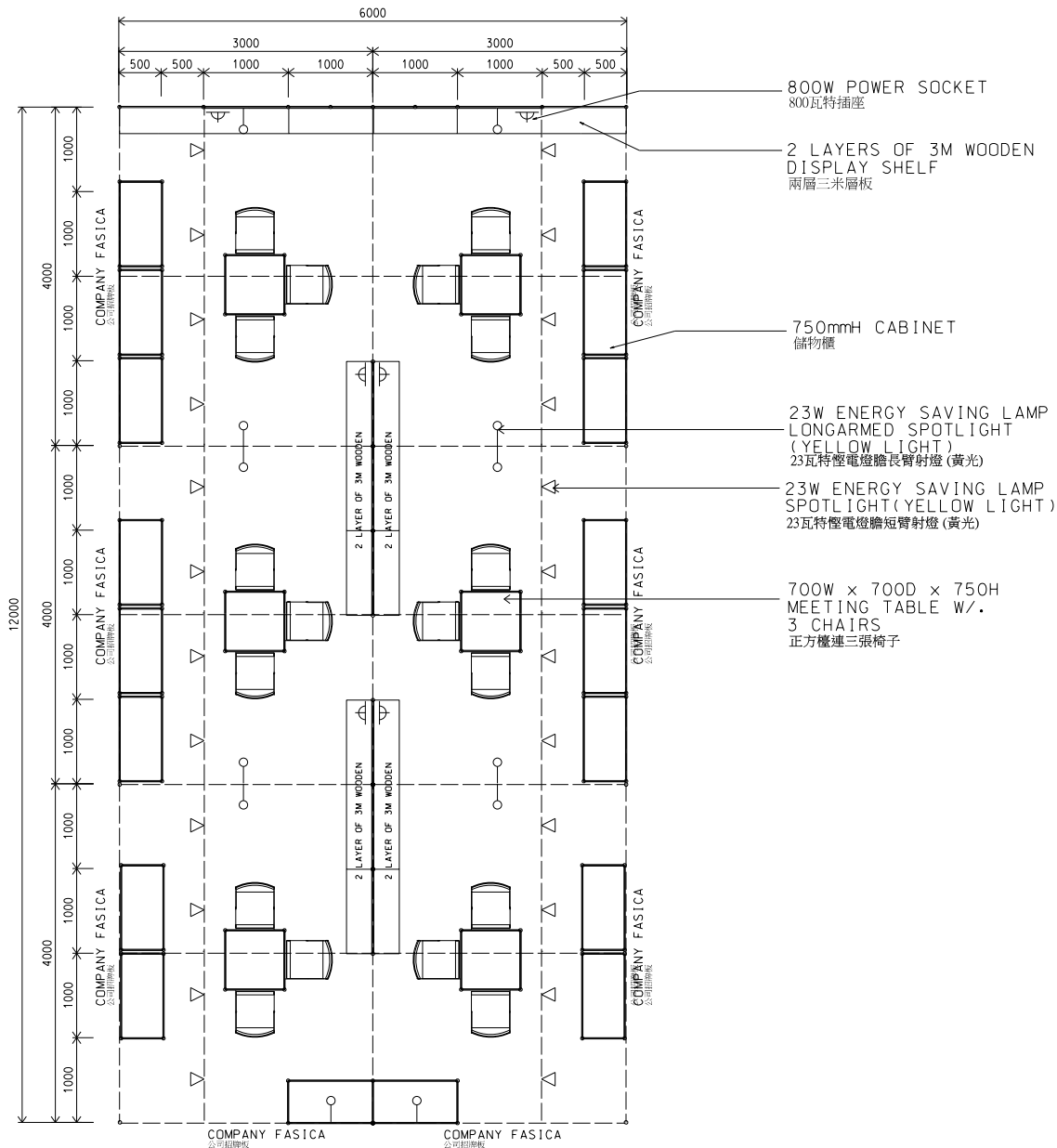
PLAN 平面圖
