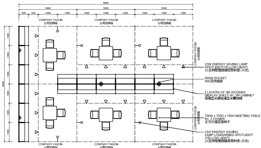
PLAN 平面圖
